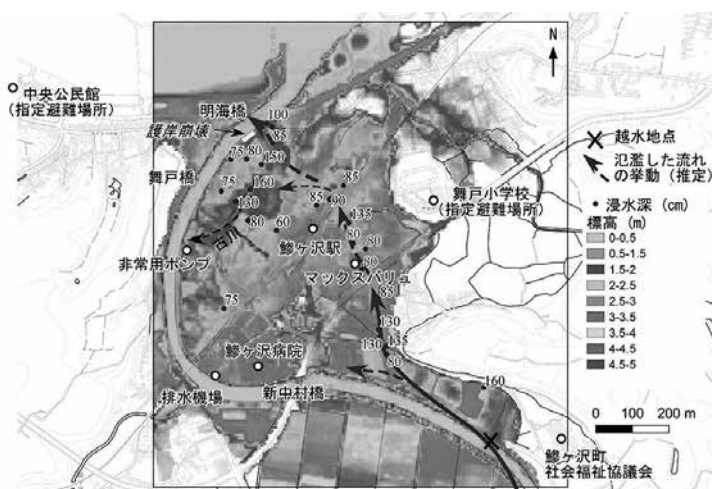
【図1】鮎ヶ沢町舞戸地区の浸水分布図（郷青類ほか「令和4年8月鮎ヶ沢町中村川の浸水被害について（速報）」 https://www.hirosaki-u.ac.jp/wp-content/uploads/2022/08/20220819.pdf ）
